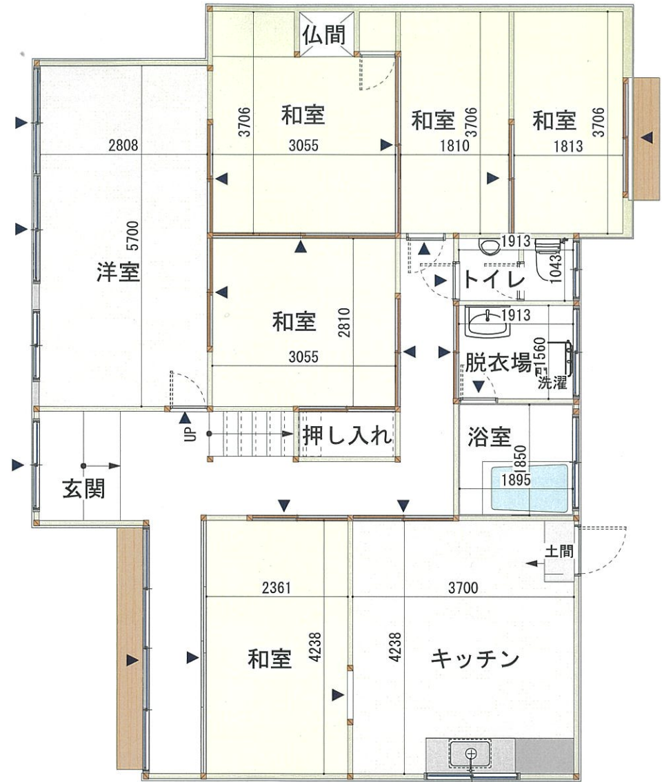
1F平面図
