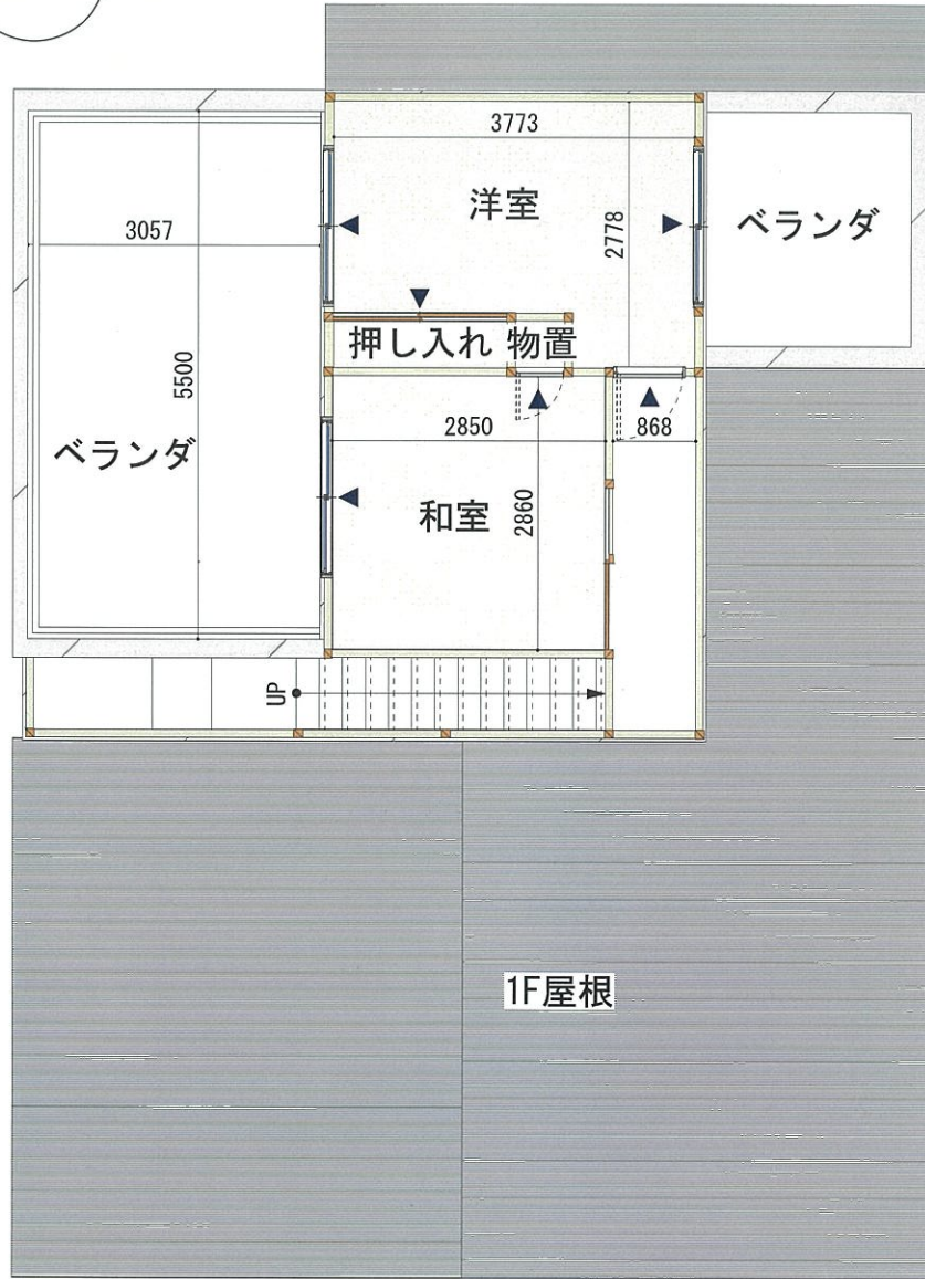
2F平面図
